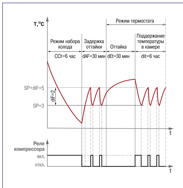
▶ Пример работы TRM974 в режиме НАБОР ХОЛОДА: график изменения температуры в камере и временная диаграмма работы реле компрессора (для значений параметров, установленных по умолчанию на заводе-изготовителе)
