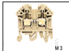
RK 2,5-4 TS 32/TS 35
